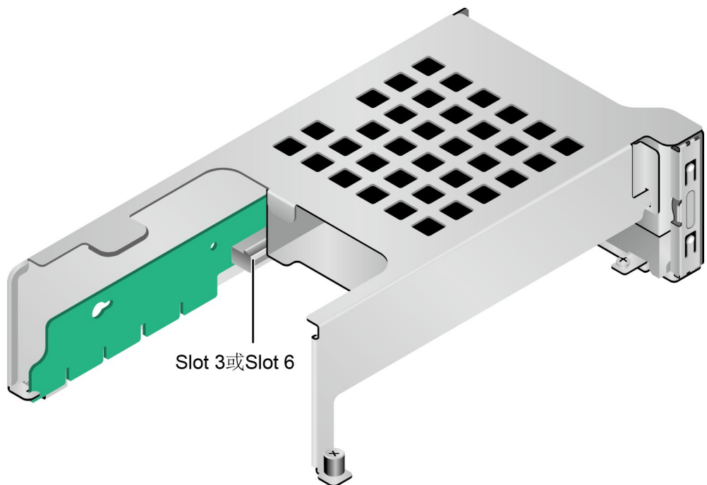
图 4-11 Riser 卡 3 (1x16)
