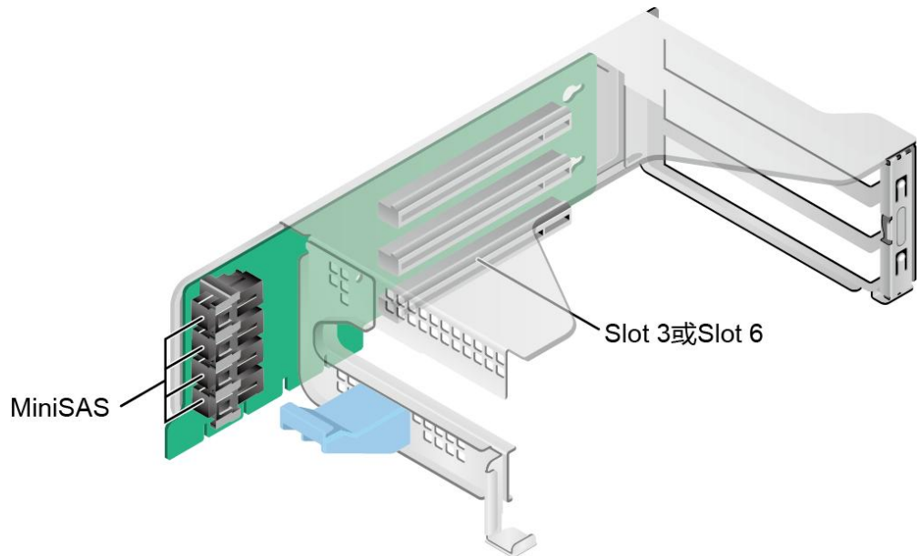
图 4-12 Riser 卡 4 (SAS Riser)
