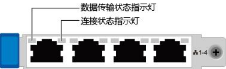
图 4-7 TM210（4*GE 电口）
