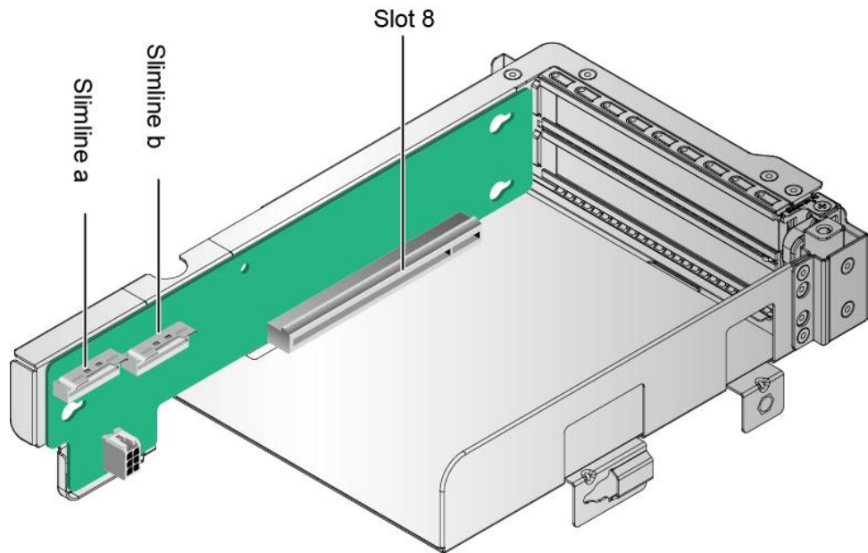
图 4-14 Riser 卡 6 (1x16)
