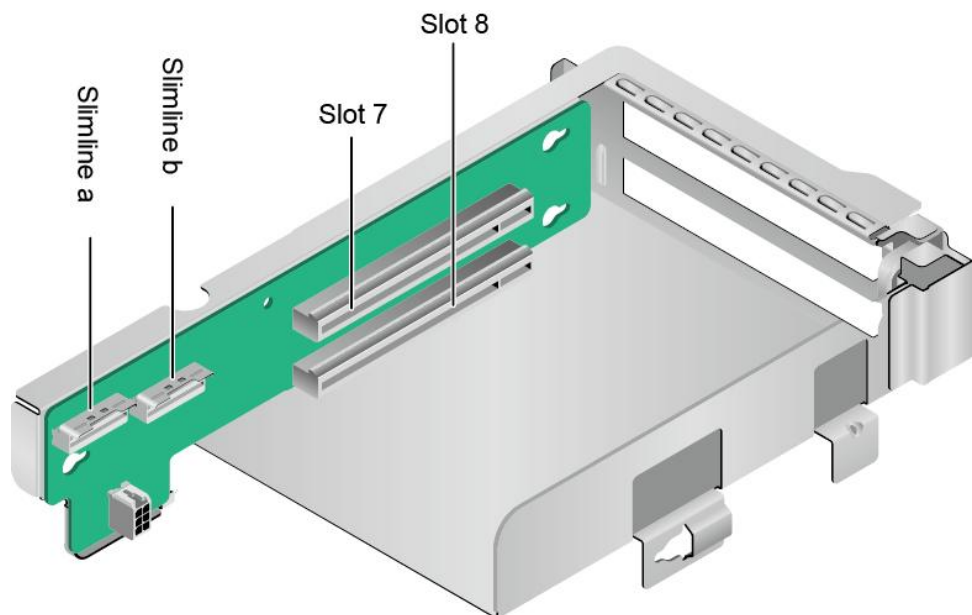
图 4-13 Riser 卡 5 (2x8)
